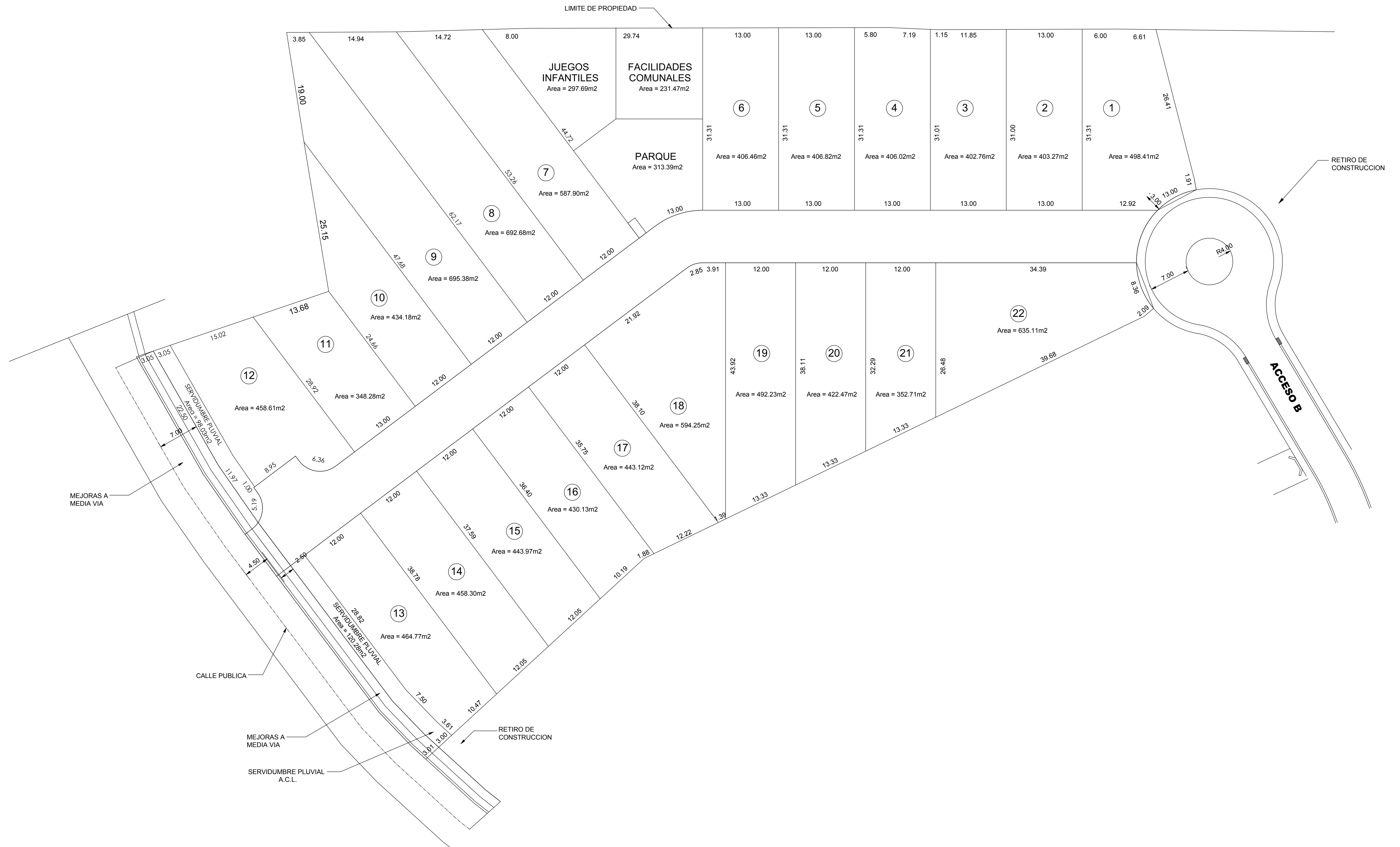
DISEÑO DE SITIO Escala: 1 : 400
